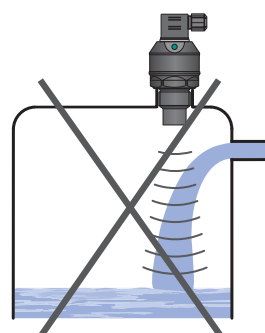
A instalação do medidor de nível deve ser feita longe do local de entrada
