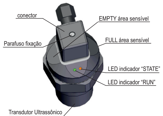
Peças principais do dispositivo de medição
