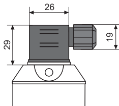
Conector DIN (G)
