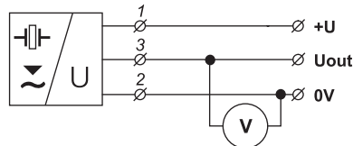
Conexão elétrica para medição de tensão (opção V) e vista interna do conector
