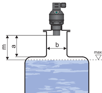
Possível instalação utilizando pescoço estendido
